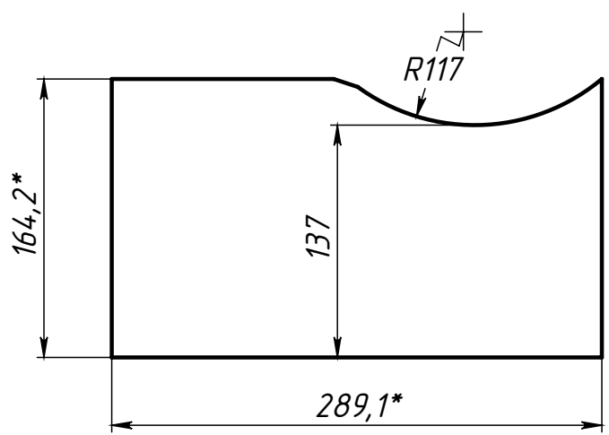
Поз.2 (Угольник)
